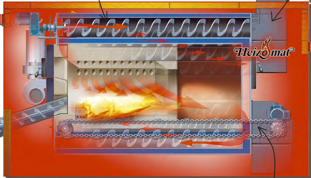
Cámara de combustión con cadenas para eliminación de cenizas
